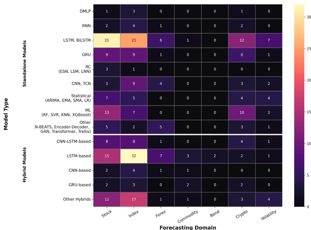
Fig. 14. Topic-Model heatmap.
